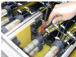
⑨ 2本目の発生器を外します。
