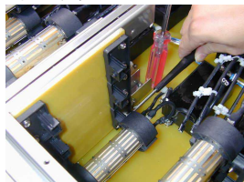
⑩ 3本目の発生器を外します。
