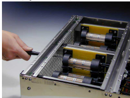
⑤ 発生器のネジを外します。
