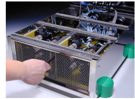
④ 発生器のネジを外します。
