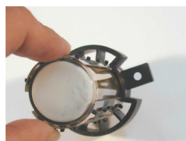
③ 電極板が正しく取り付けられているか確認します。
